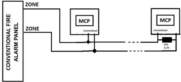
Şekil 1- KABLO BAĞLANTISI
